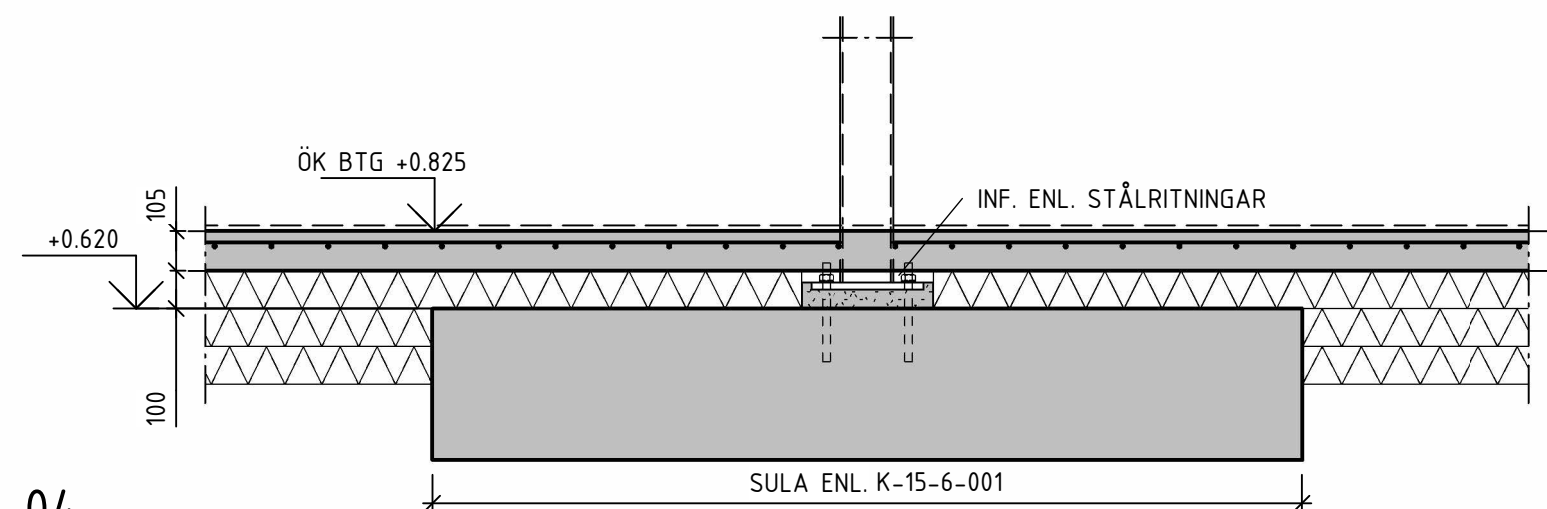
04 1 : 20 SULA UNDER GRUNDPLATTA
