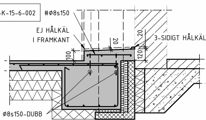
17 1 : 20 ANSLUTNING VID KULVERT MOT BEFINTLIGT FRITIDS
