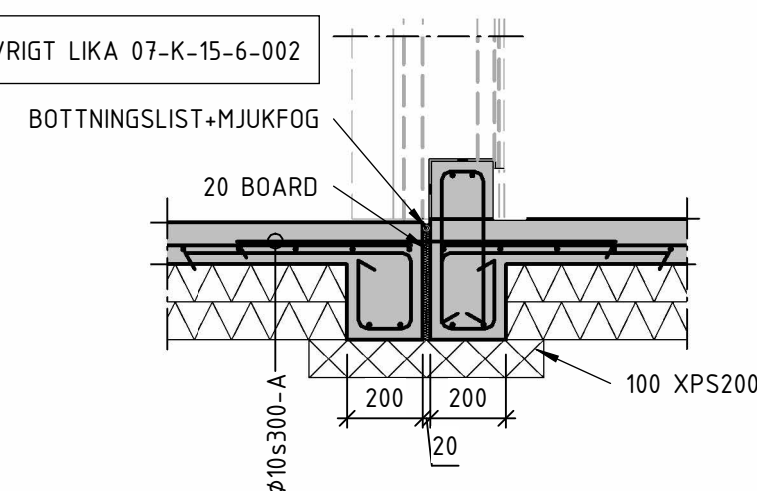
09 1 : 20 ÖVERGÅNG LASTKAJ OCH AVFALLSRUM
