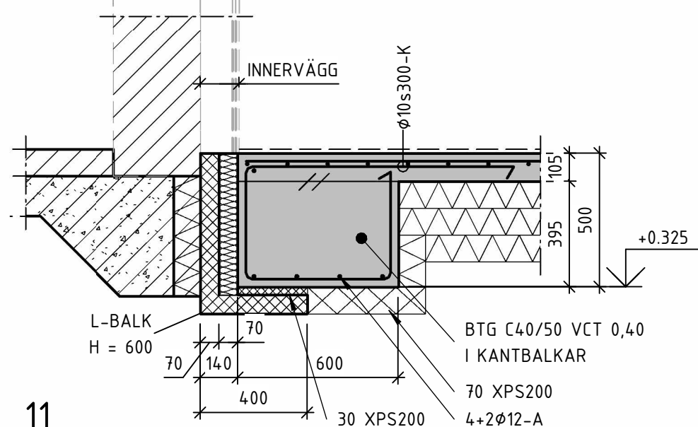
11 1 : 20 ANSLUTNING MOT BEFINTLIGT FRITIDS
