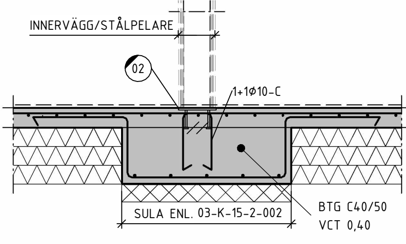
10 1 : 20 INGJUTNINGSGODS FÖR STÅLPELARE
