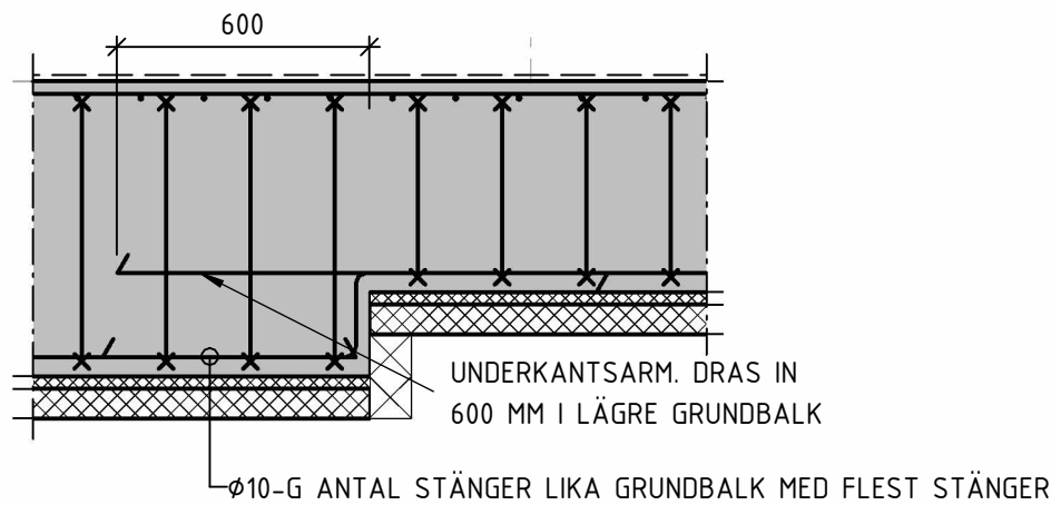
05 1 : 20 PRINCIPDETALJ ÖVERGÅNG KANTBALKSHÖJDER
