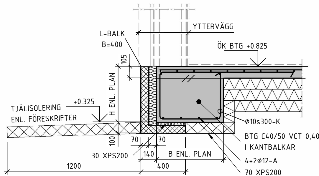
01 1 : 20 KANTBALK UNDER YTTERVÄGG
