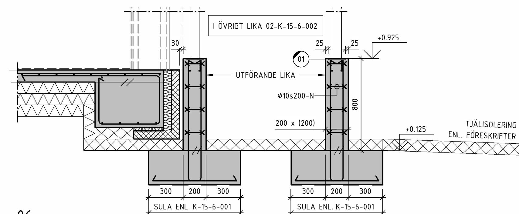
06 1 : 20 FUNDAMENT VID TRAPPA TILL FLÄKTRUM
