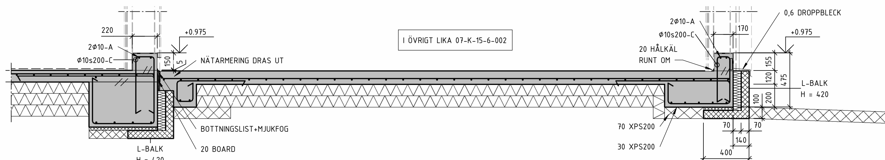
08 1 : 20 TVÄRSEKTION AVFALLSRUM
