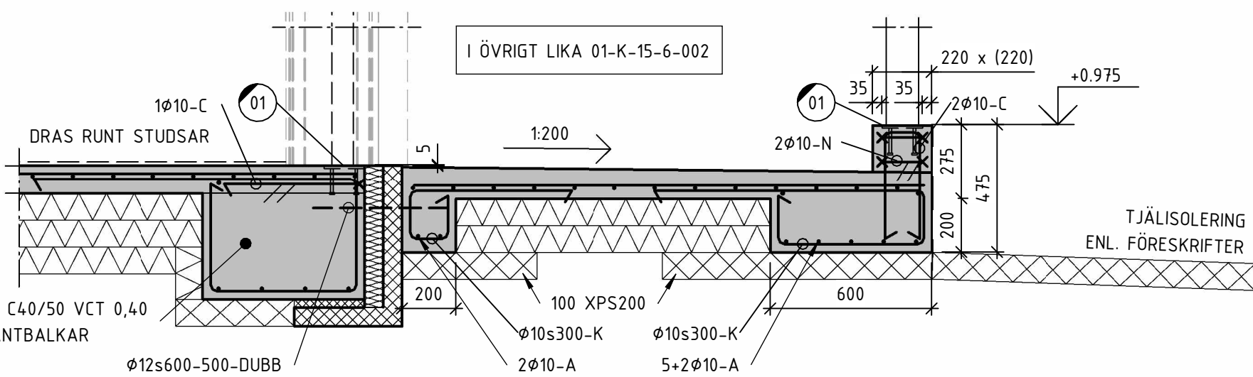
07 1 : 20 TVÄRSEKTION LASTKAJ
