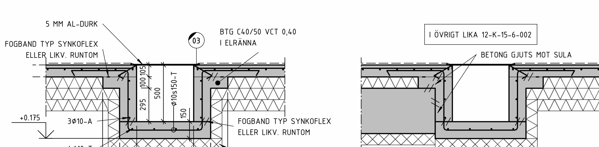
12 1 : 20 ELGROP
