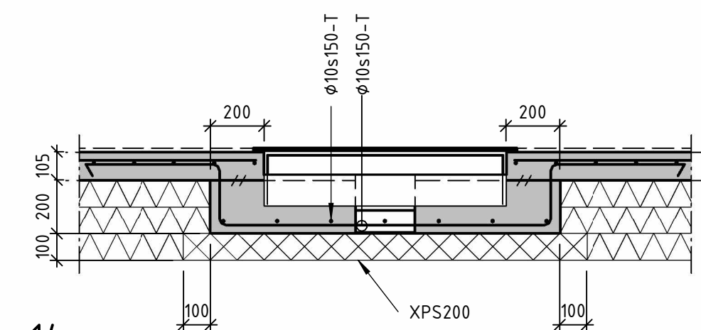
14 1 : 20 PRINCIPDETALJ AVLOPP I STORKÖK
