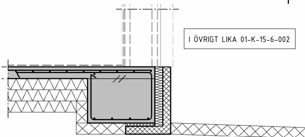
02 1 : 20 KANTBALK UNDER YTTERVÄGG
