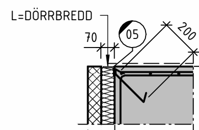
15 1 : 20 PRINCIPDETALJ L-STÅL UNDER YTTERDÖRRAR
